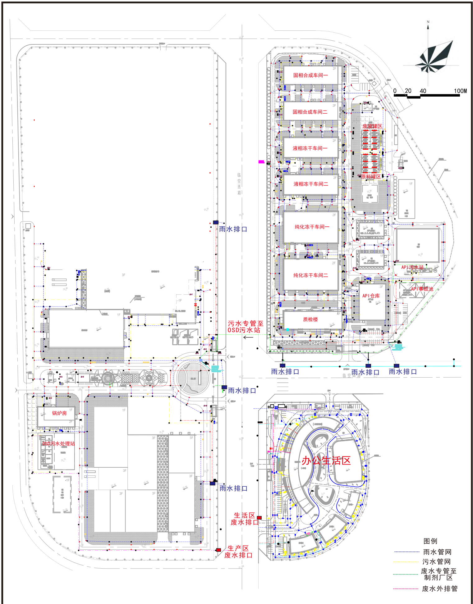
附图6 翰宇药业（武汉）有限公司生物医药生产基地 建设项目（一期）雨水、污水管网图
